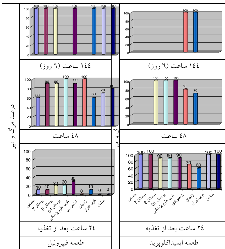
نمودار شماره ۱: مقایسه میان درصد مرگ و میر سوش حساس و سوشهای وحشی سوسری آلمانی بعد از تغذیه به مدت ۲ ساعت بر روی ژل طعمه فیپرونیل و ایمیداکلوپرید
