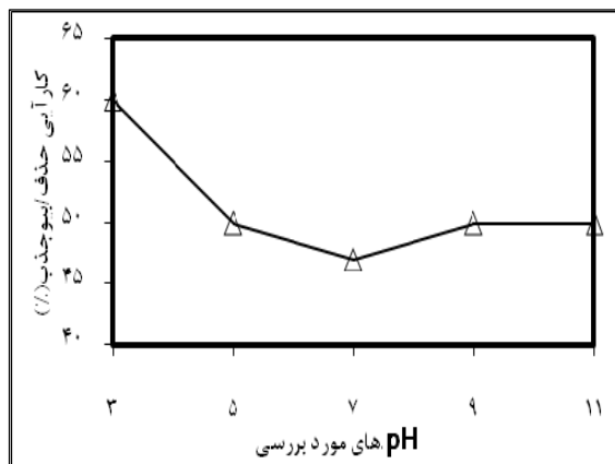
شکل ۳- نتایج بررسی اثر pH بر کارایی حذف / جذب زیستی (در غلظت ثابت رنگ، زمان تماس و دوز جاذب)
