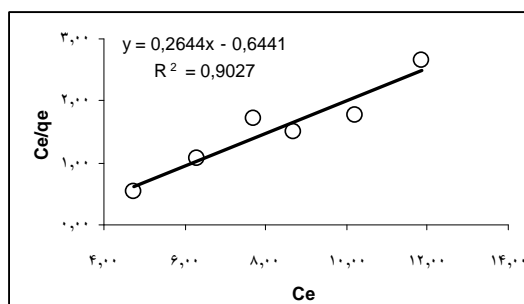
شکل ۷ ب: ایزوترم لانگموئر
