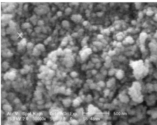
شکل ۱: تصویر الکترونی نانوذره ZnO (SEM) مجهز به سیستم Energy Dispersive X-ray (EDX) spectroscopy
